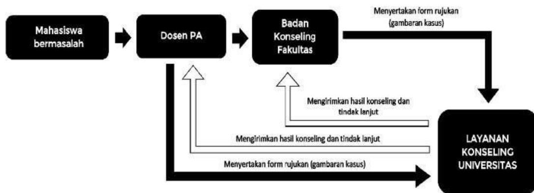
Gambar 17. Alur Rujukan
